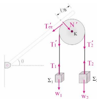
Δυνάμεις στην τροχαλία και στα σώματα \Sigma_1 και \Sigma_2
