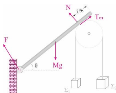
Δυνάμεις στη ράβδο
